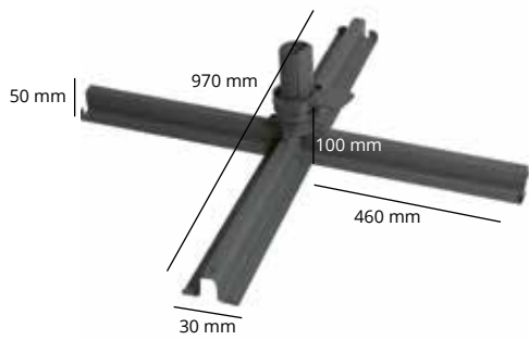
Soporte en cruz
