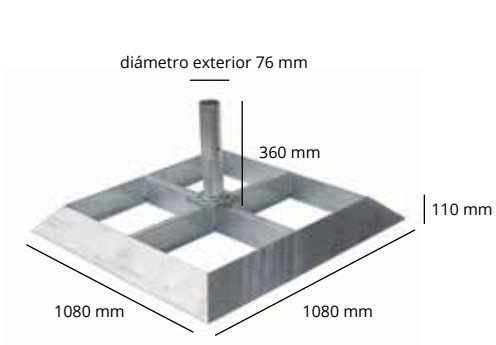
Soporte de baldosas
