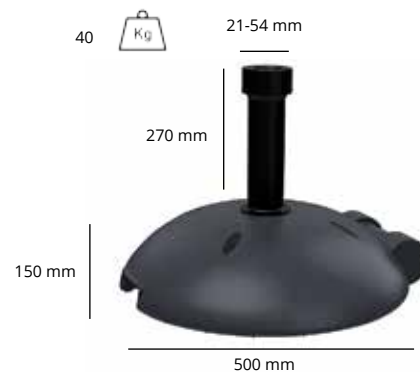
Base de hormigón cubierta de resina
